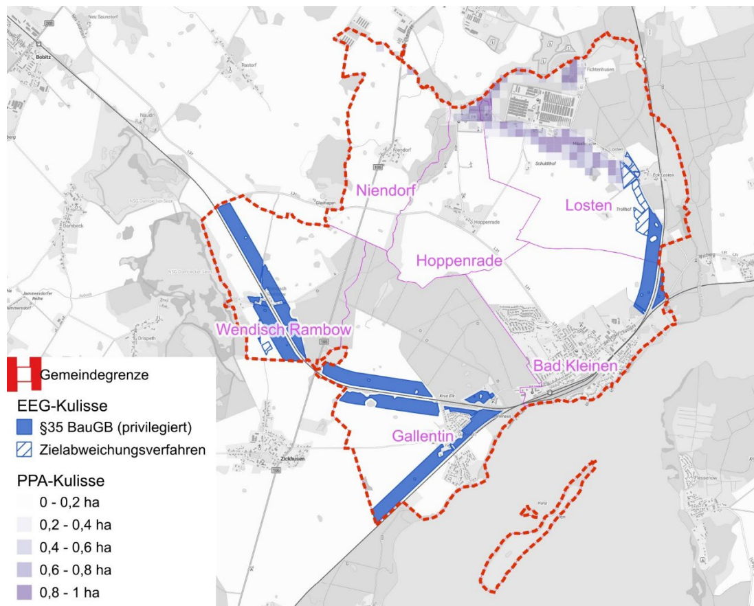
Abbildung 20: Räumliche Ergebnisdarstellung zum Photovoltaik-Flächenanlagenpotenzial
